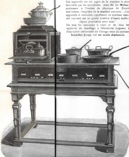
Tischherd, 4 Platten, 1 Backofen. Four à cuire et à rôtir, avec quatre plats.
